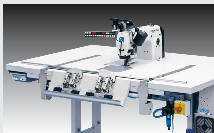
Beisler 739-23-01 – CNC-gesteuerte Nähanlage mit Doppelsteppstich zum Vornähen und Beschneiden von Manschetten (~ 1.800 Manschetten in 480')
